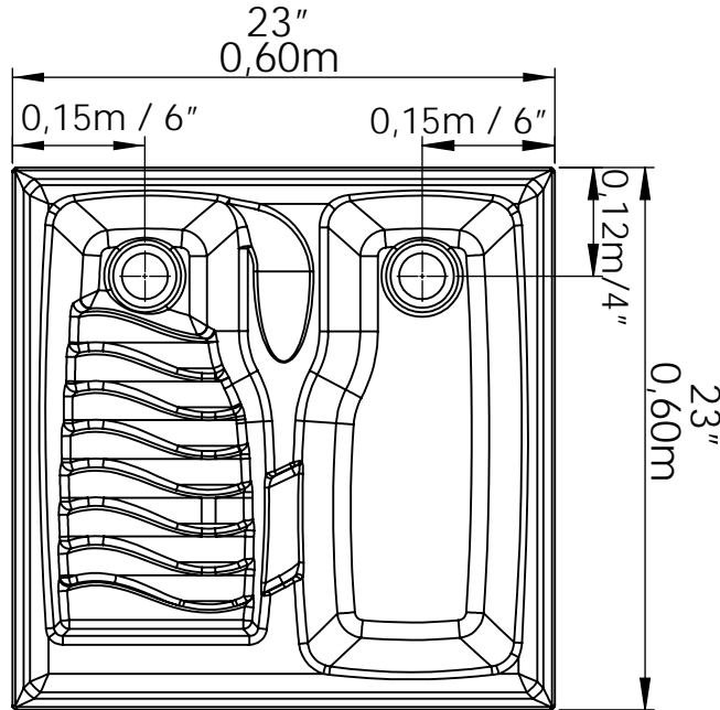
VISTA EN PLANTA / PLANT VIEW
