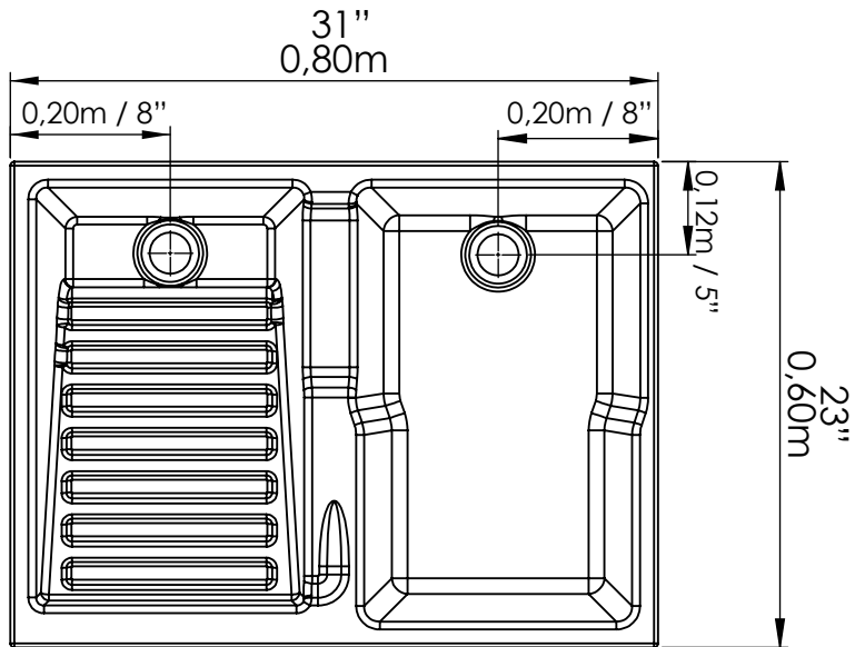
VISTA EN PLANTA / PLANT VIEW
