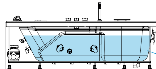
llenado de hidromasaje Hydromassage filling
